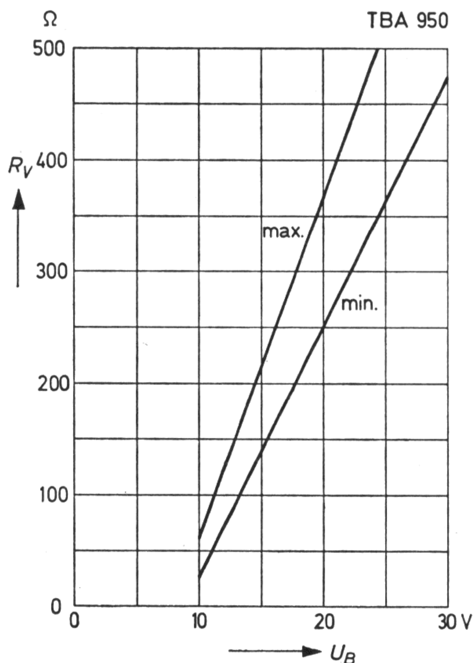
Bild 8: Diagramm zur Ermittlung des Vorwiderstandes R_V .
