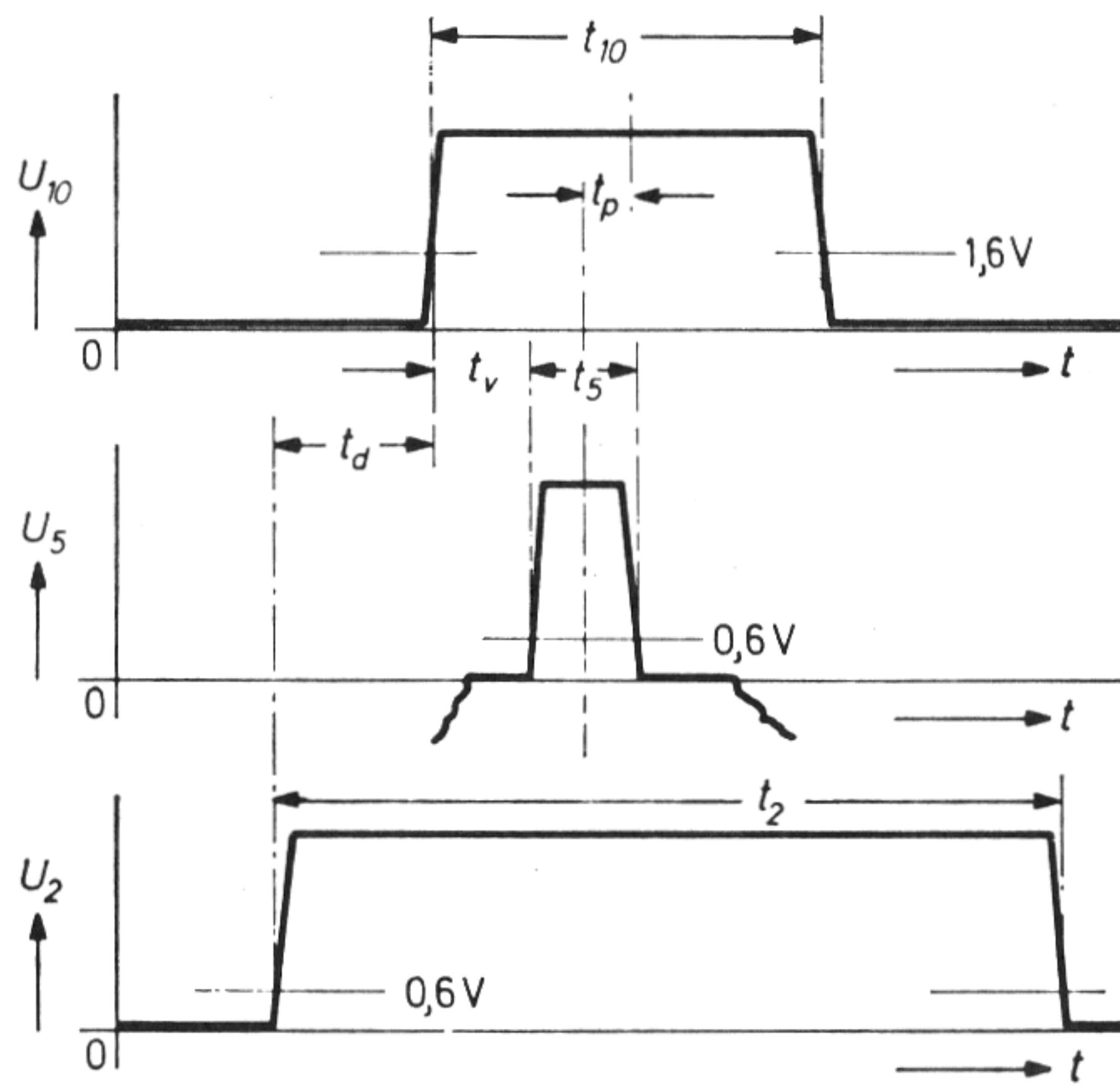
Bild 4: Phasenbeziehungen beim TBA 950.
