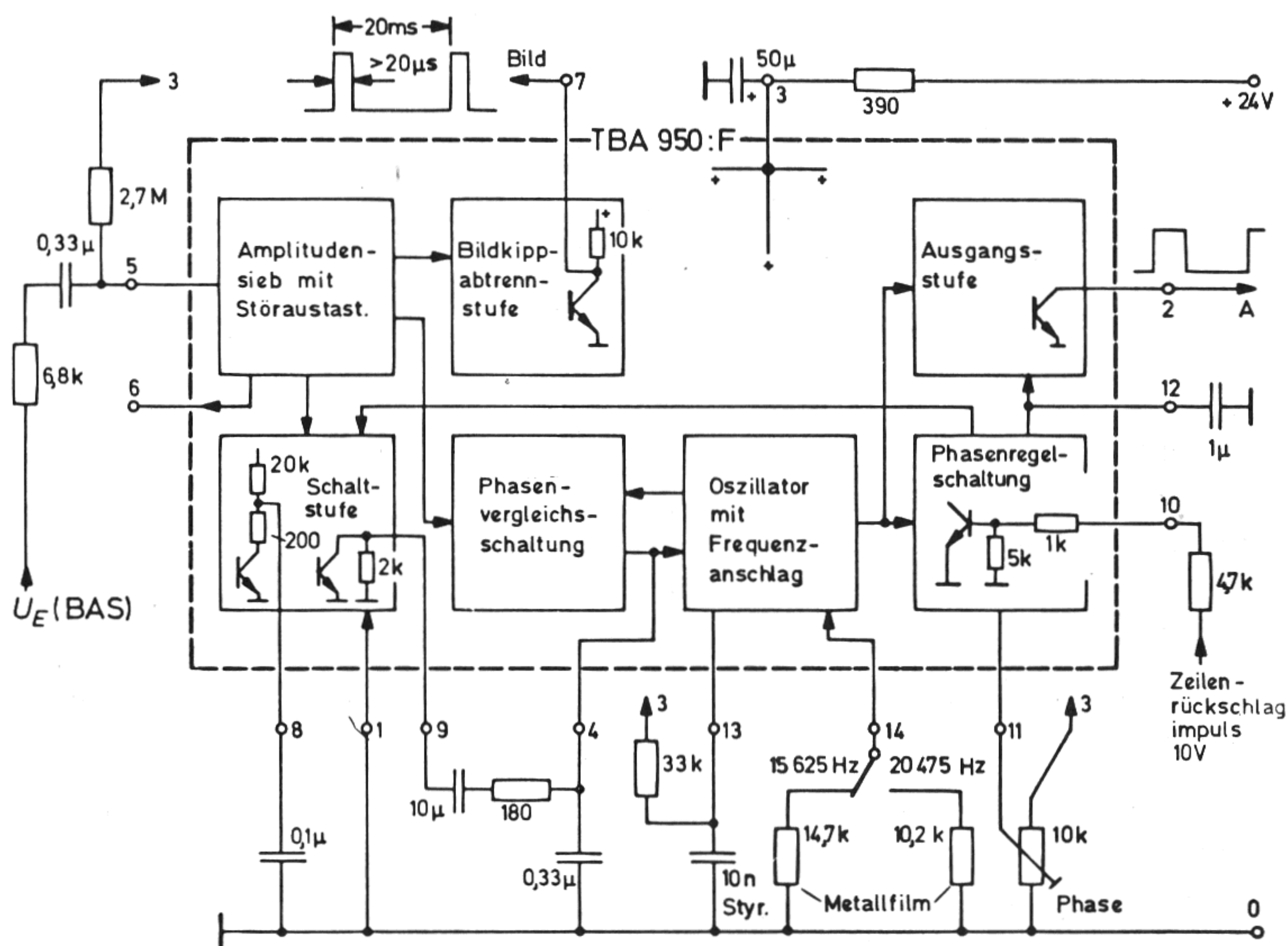
Bild 3: Blockschaltbild des TBA 950:F und Meßschaltung für die Kennwerte.
