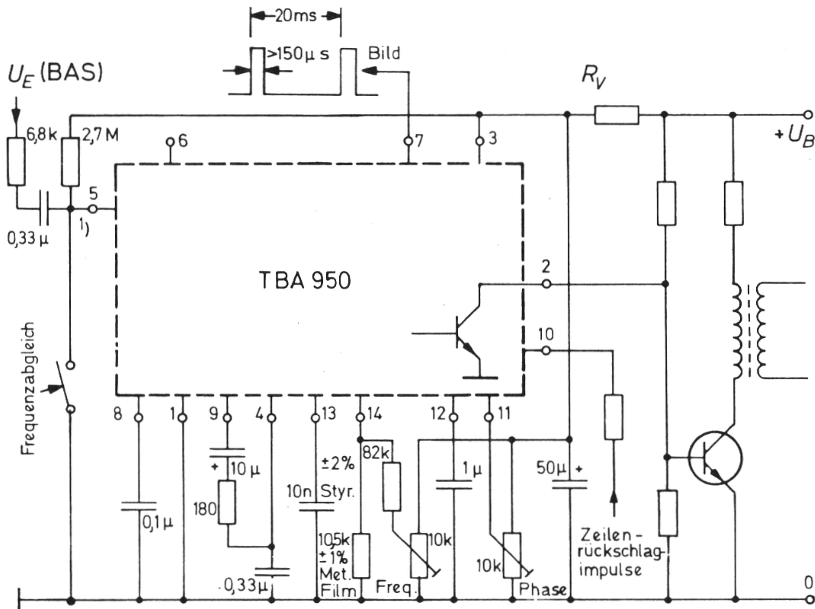
Bild 6: Betriebsschaltung des TBA 950, Alternativvorschlag zur Frequenzeinstellung
