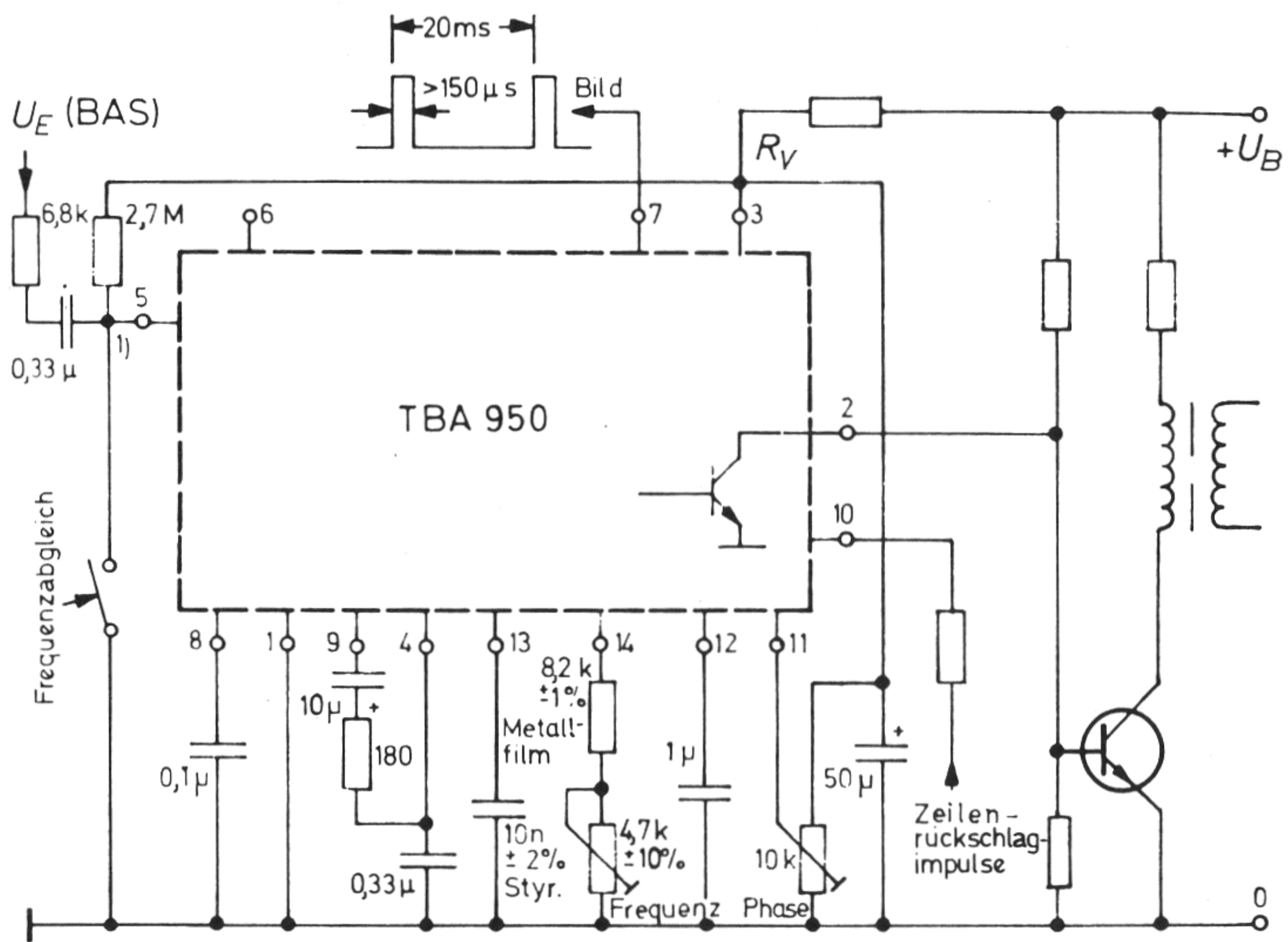
Bild 5: Betriebssystem des TBA 950 1) Eingangsschaltung im Empfänger optimieren
