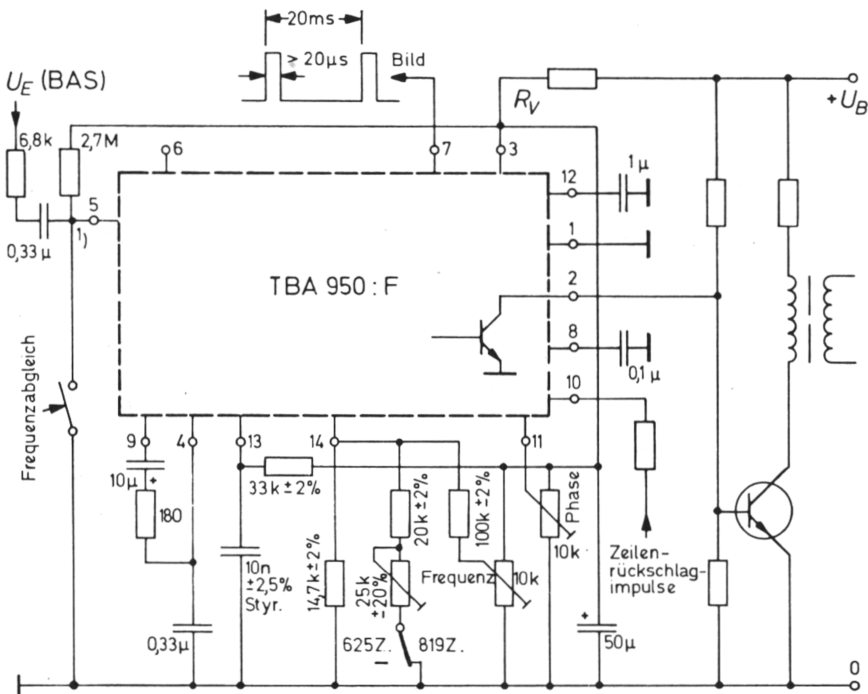
Bild 7: Betriebsschaltung des TBA 950:F mit Umschaltung von 625 Zeilen auf 819 Zeilen
